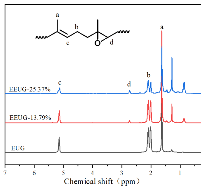
图 1 杜仲胶(EUG)和环氧杜仲胶(EEUG)核磁谱图 ( ^1\text{H} -NMR)
