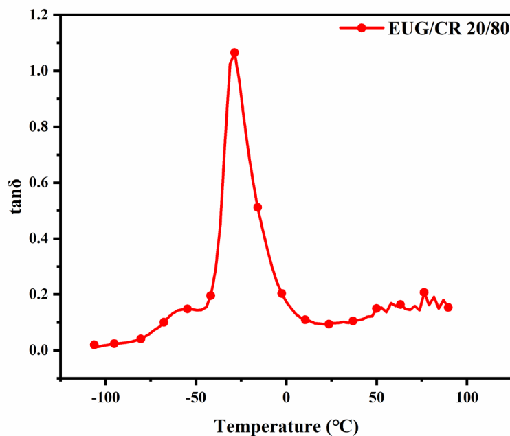
图 9 共混杜仲胶（EUG/CR 20/80）的损耗因子图
