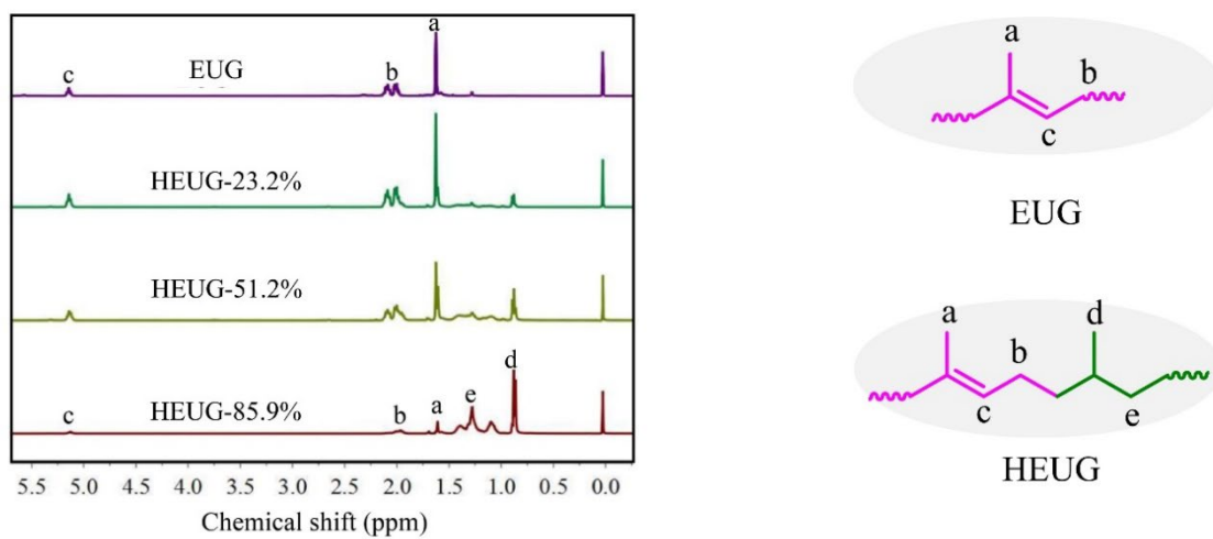
图 2 杜仲胶(EUG)和氢化杜仲胶(HEUG)核磁谱图 ( ^1\text{H} -NMR)
