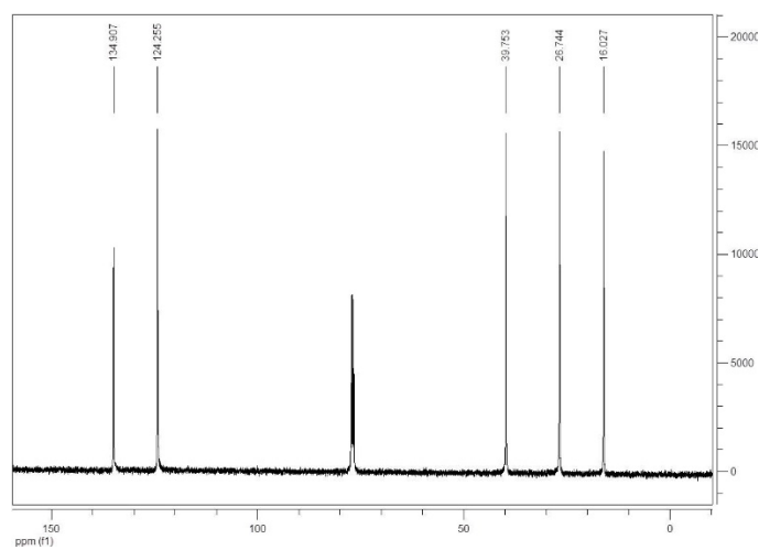
图 4 杜仲胶核磁碳谱谱图 ( ^{13}\text{C} -NMR)
